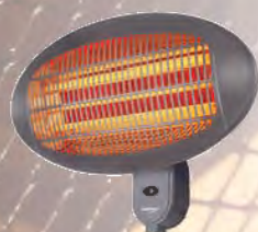
Calefactor eléctrico mural Habitex E398 3 potencias: 650/1.300/2.000 W. Para acoplar directamente sobre pared. Protección contra salpicaduras IPX4. 50x18xh.36 cm. 9310R398
